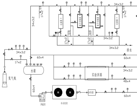
图 1 CSNS 靶站水冷却系统实验平台
