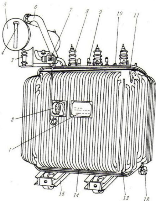
1.铭牌；2.信号式温度计；3.吸湿器；4.油标；5.储油柜；6.安全气道 7.气体继电器；8.高压套管；9.低压套管；10.分接开关；11.油箱；12. 放油阀门；13.器身；14.接地板；15.小车
