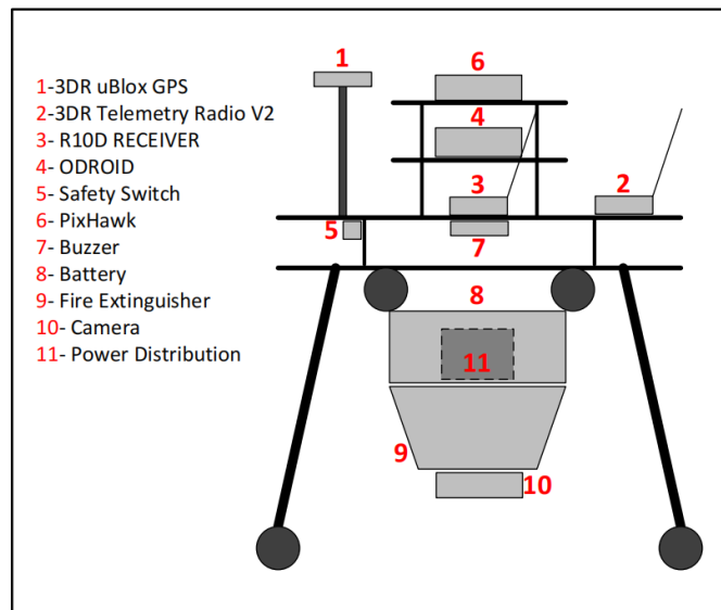
图 6 FXUAV 的结构
